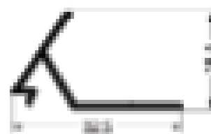
2581 Jerguilla extra cóncava (20mm) Peso: 0.182 kg/m
