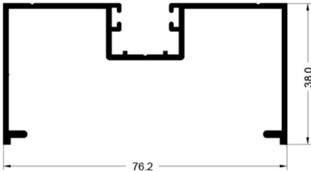
1161 Perimetral fijo Peso: 0.828 kg/m
