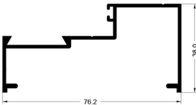
1163 Perimetral móvil Peso: 0.730 kg/m
