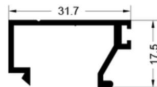
1164 Junquillo Peso: 0.296 kg/m
