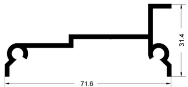
3103 Ancla Peso: 0.720 kg/m
