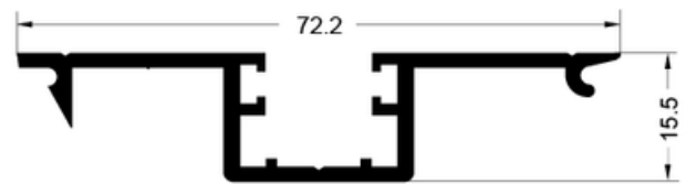
1162 Tapa acanalada Peso: 0.604 kg/m
