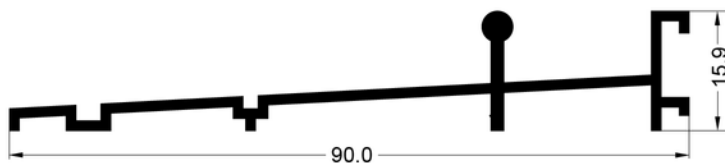
1111 Riel inferior Peso: 0.551 kg/m
