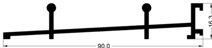
1452 Riel inferior doble Peso: 0.750 kg/m
