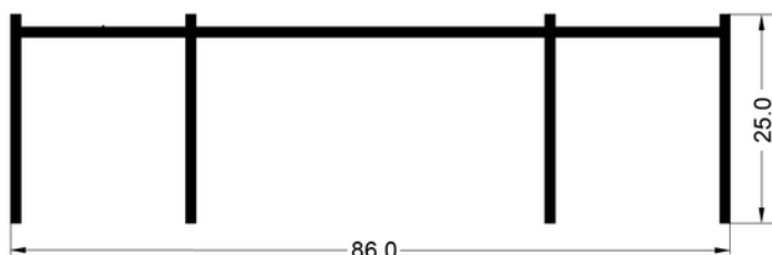
1110 Riel superior Peso: 0.637 kg/m
