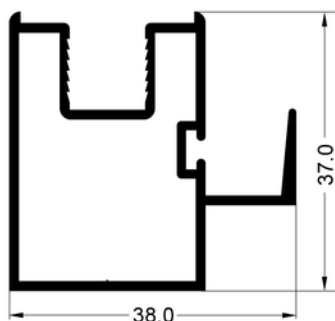
1108 Entrecierre Peso: 0.604 kg/m
