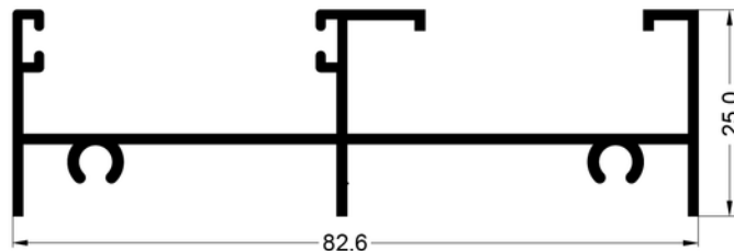
1109 Jamba marco Peso: 0.727 kg/m
