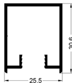
1116 Vertical de hoja Peso: 0.421 kg/m
