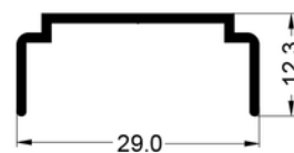
1059 Adaptador Peso: 0.167 kg/m
