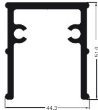
1342 Ancla Peso: 1.496 kg/m
