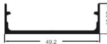
1345 Contratapa pequeña Peso: 0.361 kg/m
