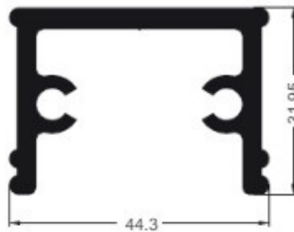
1343 Ancla pequeña Peso: 1.156 kg/m
