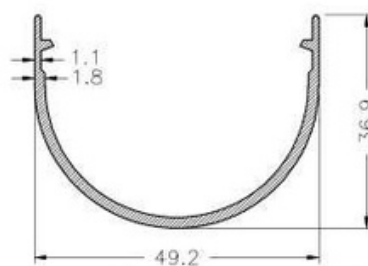
1344 Contratapa grande Peso: 0.565 kg/m
