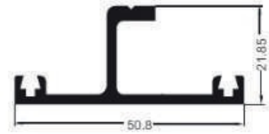
1338 Espalda falsa Peso: 0.576 kg/m
