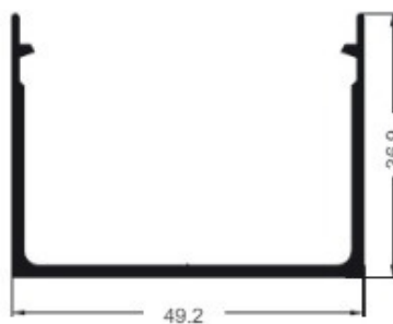
1344 Contratapa grande Peso: 0.565 kg/m
