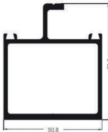
1337 Espalda pequeña Peso: 1.415 kg/m
