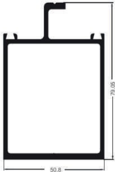
1336 Espalda Peso: 1.643 kg/m
