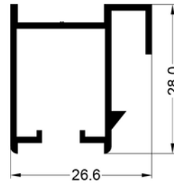
2232 Entrecierre fijo Peso: 0.342 kg/m
