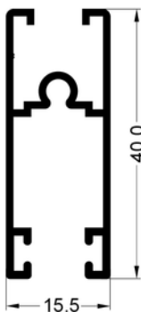
2233 Horizontal de hoja Peso: 0.388 kg/m
