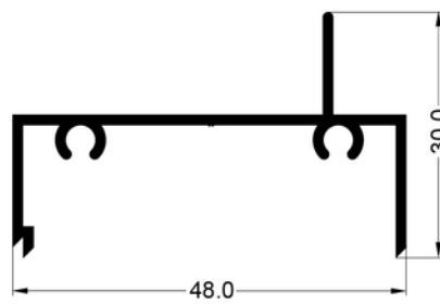
2234 Jamba marco Peso: 0.393 kg/m
