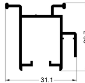
2235 Entrecierre móvil Peso: 0.378 kg/m
