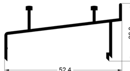
2238 Riel inferior Peso: 0.392 kg/m
