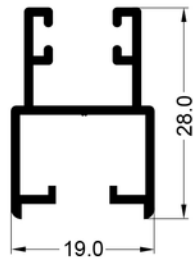
2231 Vertical de hoja Peso: 0.322 kg/m
